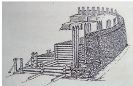
Velkomoravská hradba v Rybárnách, jak ji podle výsledků výzkumu nakreslil archeolog Luděk Galuška. Kresba: Luděk Galuška
