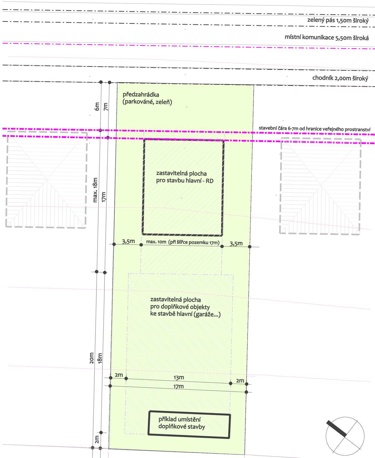
Odstupové vzdálenosti u pozemku 17m x 44m
